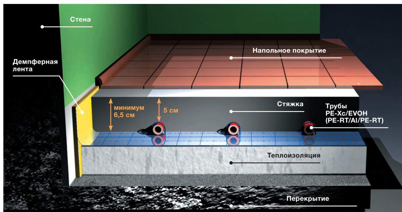
Структура пола в разрезе
