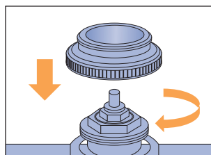
Монтаж
