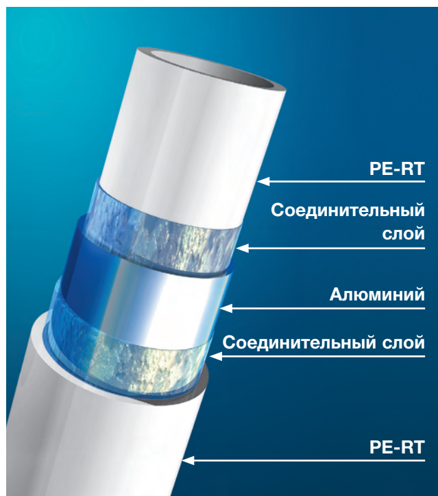
Труба PE-RT/Al/PE-RT
